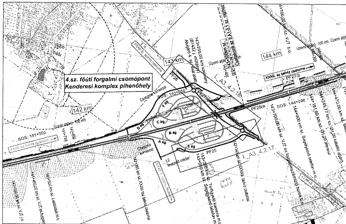
Átnézeti helyszínrajz.
