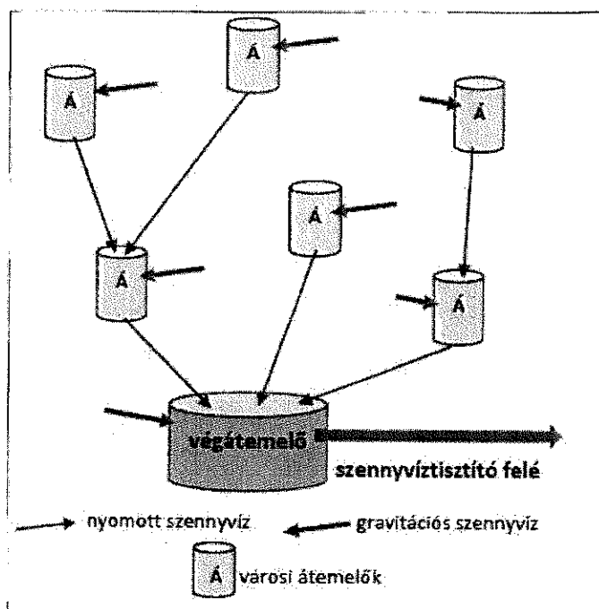
24. ábra. Szennyvíz összegyűjtése és kijuttatása a tisztítótelepre
