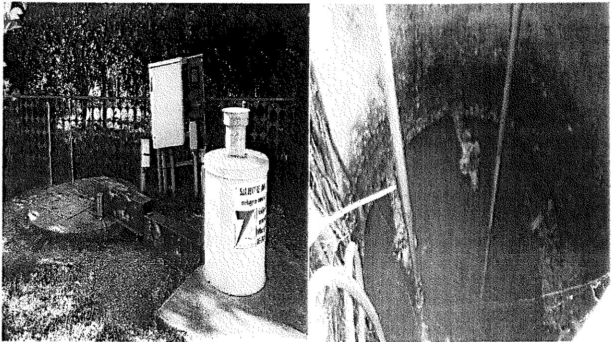
29. ábra. Rövid utcai átemelő
