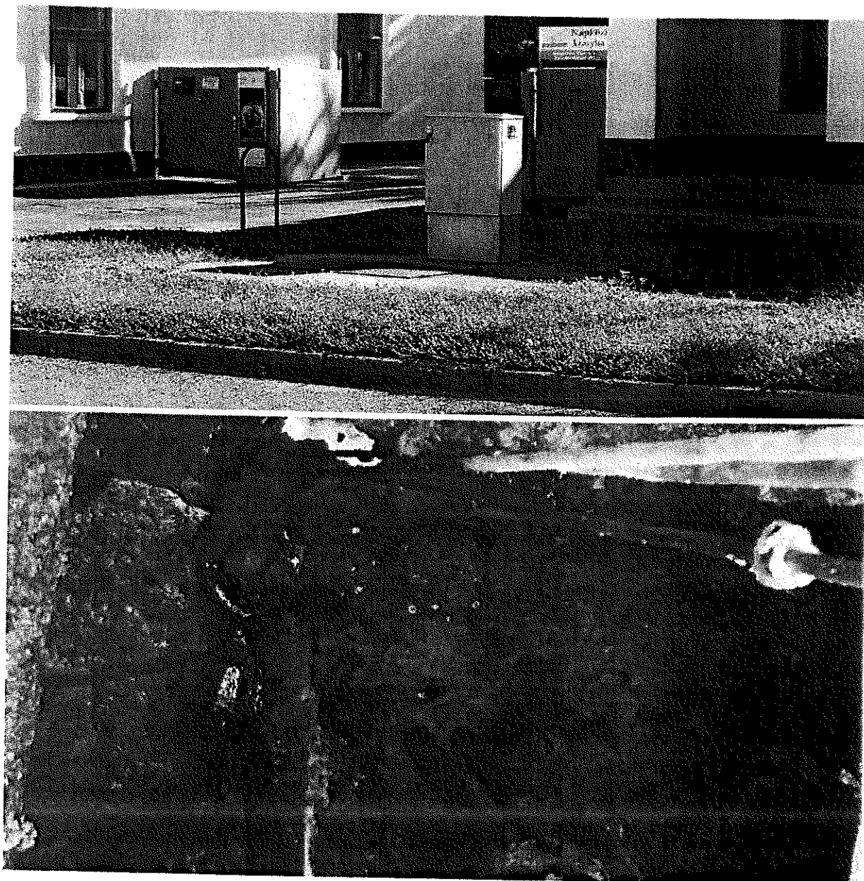
32. ábra. Vásár utcai átemelő
