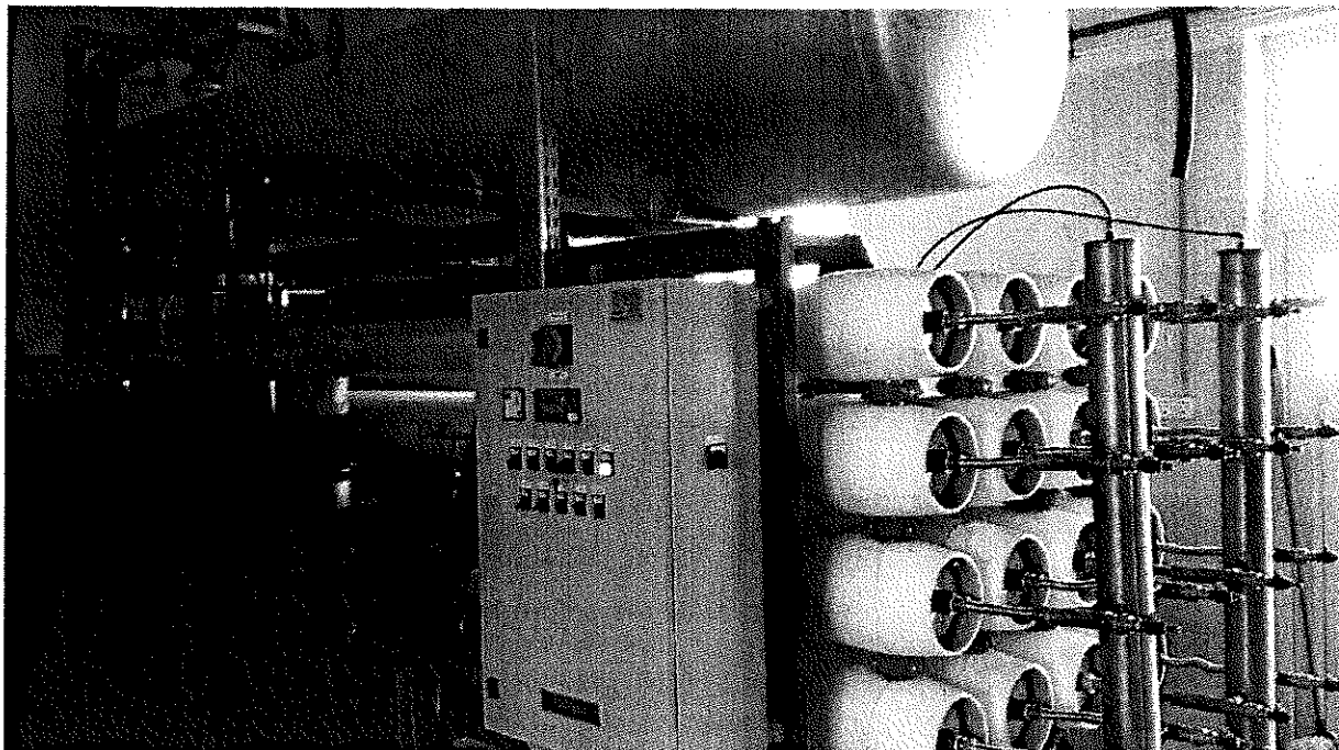
2. ábra. Szűrőberendezések
