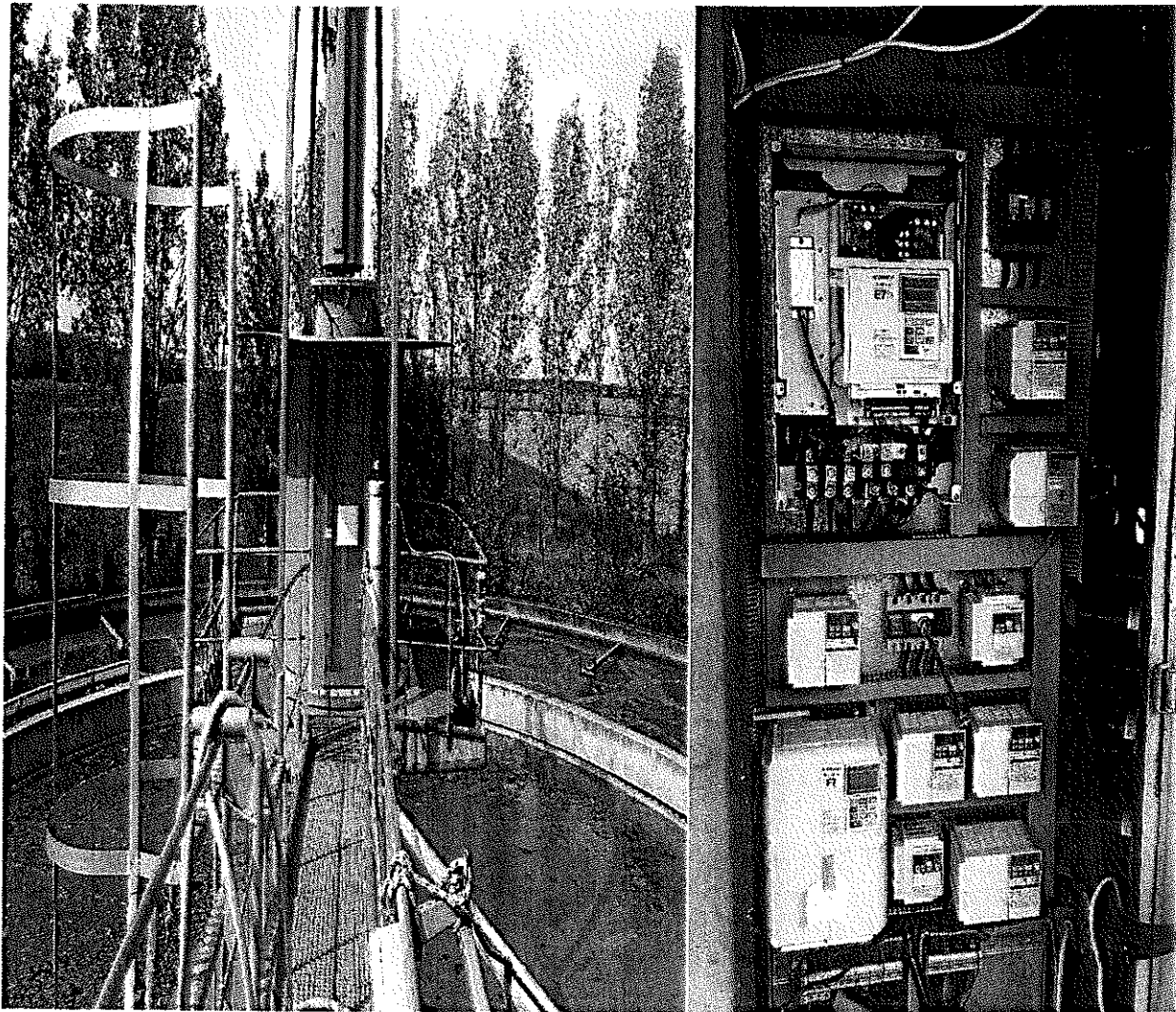
21. ábra. Kotróhid törzse és benn a légfúvó frekvenciaváltója
