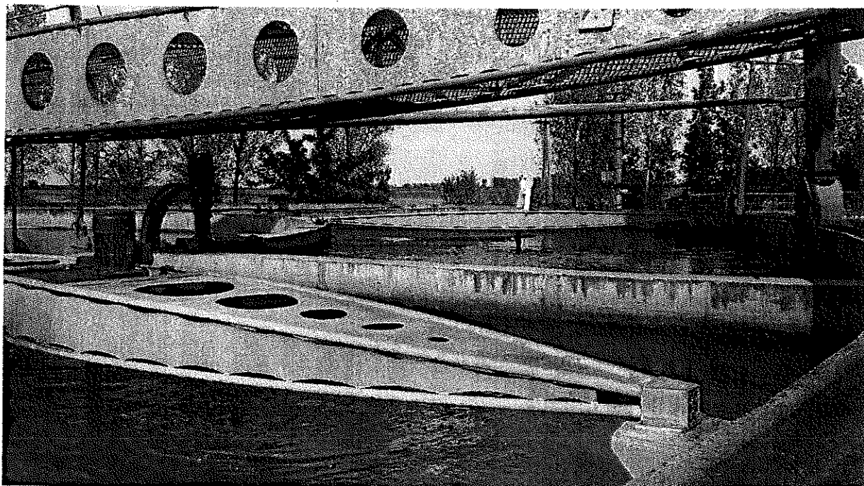
19. ábra. Anaerob és anoxikus medence kotróhídja
