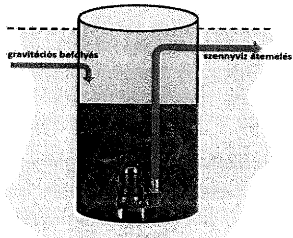
23. ábra. Gyűjtőakna szemléltetése átemelő szivattyúval
